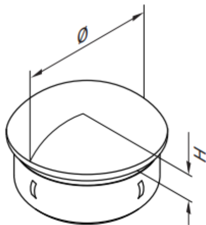
Tapa final semiesférica - estampación
