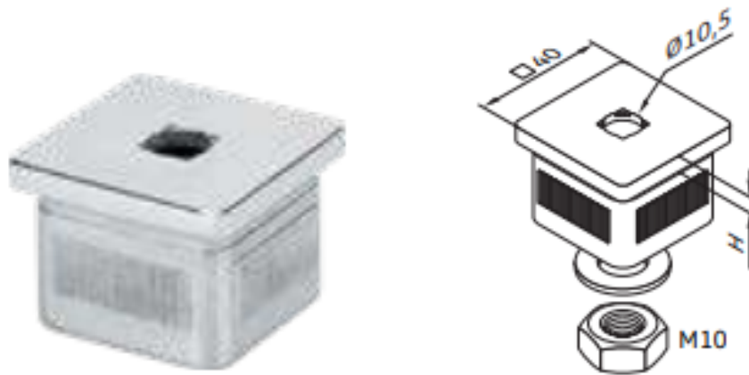
Tapón cuadrada 40 x 40 con rosca M10
