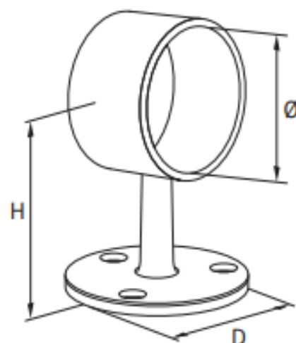
Soporte para pasamanos - fijación a pared
