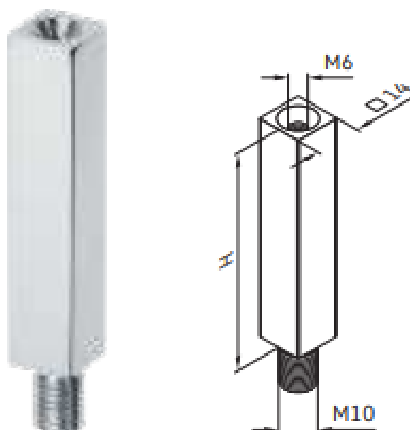
Pin cuadrado con rosca M10
