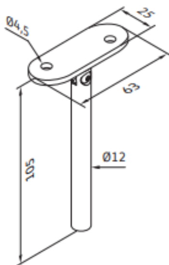
Soporte vertical para tubo plano - (regulable)
