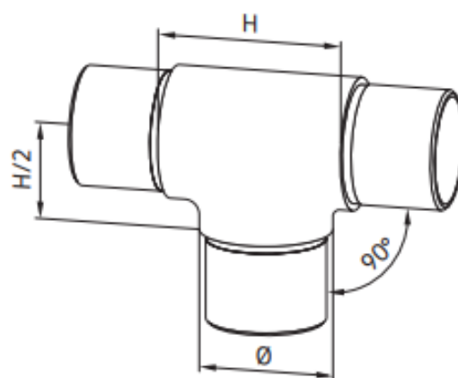
Conector para 3 tubos
