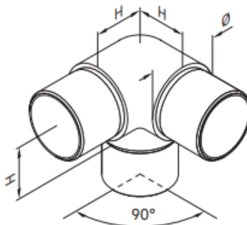
Conector para 3 tubos
