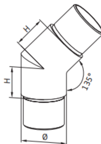
Codo conector 135° para 2 tubos
