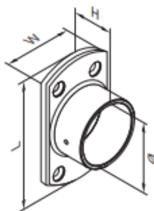
Soporte para tubo redondo - fijación a pared
