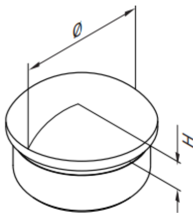
Tapa final semiesférica - fundición
