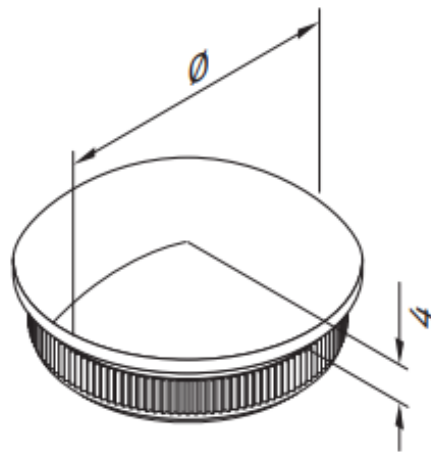
Tapa final semiesférica - fundición
