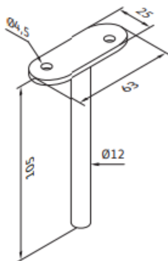
Soporte vertical para tubo plano
