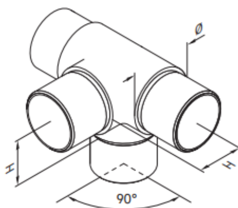
Conector para 4 tubos
