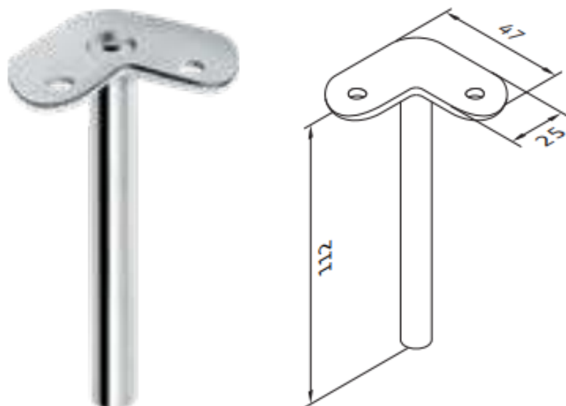
Soporte vertical 90° para tubo redondo
