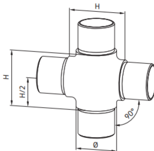
Conector para 4 tubos
