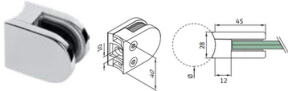
Prensacristal 45 x 40 x 28 - fijación a tubo redondo
