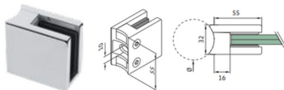
Prensacristal 55 x 55 x 32 - fijación a tubo redondo con placa de seguridad
