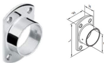
Soporte para tubo redondo - fijación a pared
