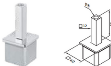
Soporte para pasamanos con rosca M8
