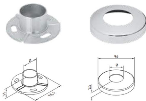
Base para tubo redondo - fijación a suelo
