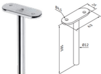
Soporte vertical para tubo plano
