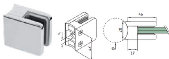
Prensacristal 46 x 45 x 28 - fijación a tubo redondo
