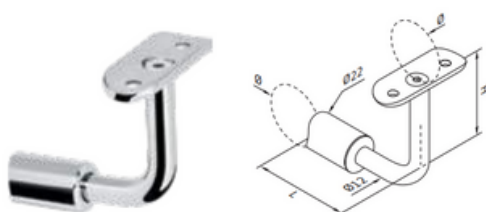
Soporte para pasamanos - fijación a tubo
