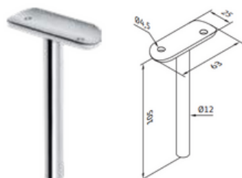
Soporte vertical para tubo redondo
