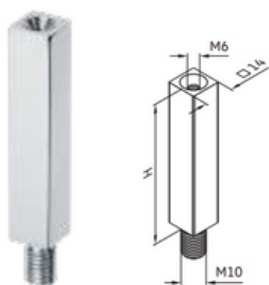
Pin cuadrado con rosca M10
