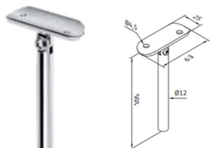
Soporte vertical para tubo redondo - regulable
