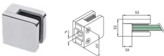
Prensacristal 55 x 55 x 32 - fijación a tubo plano
