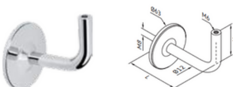
Soporte para pasamanos con rosca M6 - fijación a pared solo varilla
