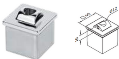
Conector a tubo para soporte vertical
