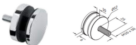
Adaptador para vidrio - fijación a pared
