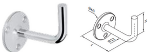
Soporte para pasamanos - fijación a pared
