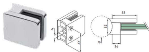
Prensacristal 55 x 55 x 32 - fijación a tubo redondo
