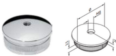
Tapa final con taladro rosca M8
