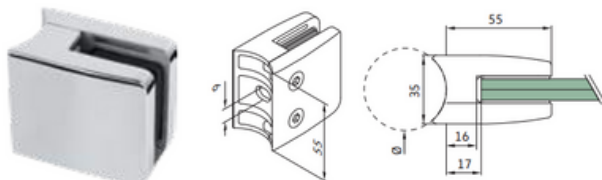
Prensacristal 55 x 55 x 35 - fijación a tubo redondo con placa de seguridad
