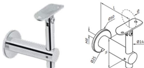
Soporte para pasamanos - fijación a pared - regulable ↕
