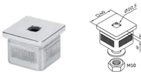
Tapón cuadrada 40 x 40 con rosca M10
