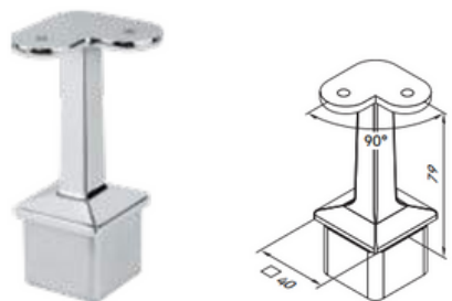
Soporte pasamano 90° de tubo plano
