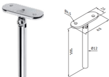
Soporte vertical para tubo plano - regulable
