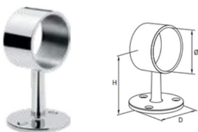
Soporte para pasamanos - fijación a pared central
