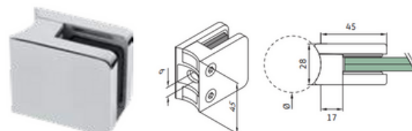
Prensacristal 45 x 45 x 28 - fijación a tubo redondo
