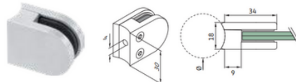
Prensacristal 34 x 30 x 18 - AISI 304 Satinado fijación a tubo redondo
