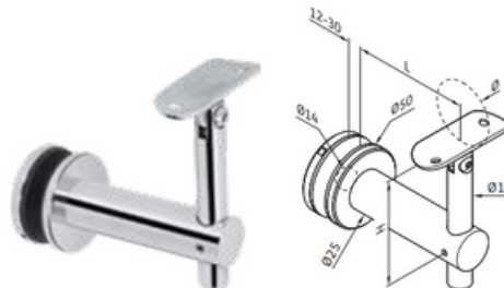
Soporte para pasamanos - fijación a cristal - regulable ↕
