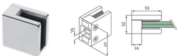
Prensacristal 55 x 55 x 32 - fijación a tubo plano con placa de seguridad
