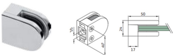
Prensacristal 50 x 40 x 24 - fijación a tubo plano
