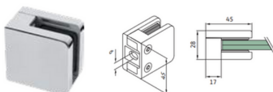
Prensacristal 45 x 45 x 28 - fijación a tubo plano
