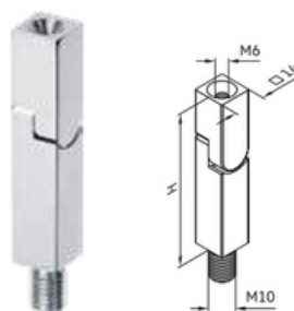
Pin cuadrado con rosca M10 - regulable
