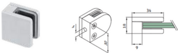
Prensacristal 34 x 30 x 18 - AISI 304 Satinado fijación a tubo plano
