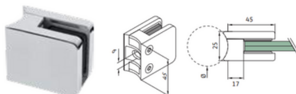
Prensacristal 45 x 45 x 25 - fijación a tubo redondo
