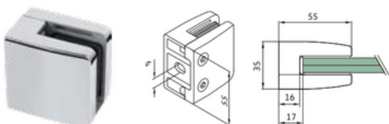
Prensacristal 55 x 55 x 35 - fijación a tubo plano con placa de seguridad
