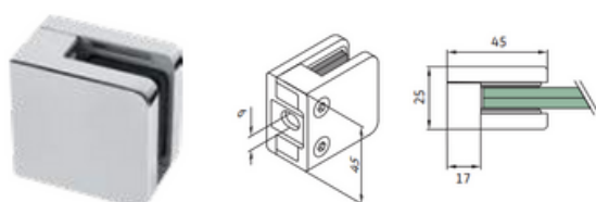
Prensacristal 45 x 45 x 25 - fijación a tubo plano
