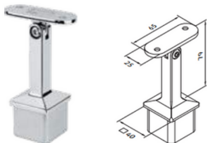
Soporte pasamano de tubo plano - regulable
