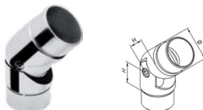
Codo conector para 2 tubos - regulable ↻ a 90° - 180°
